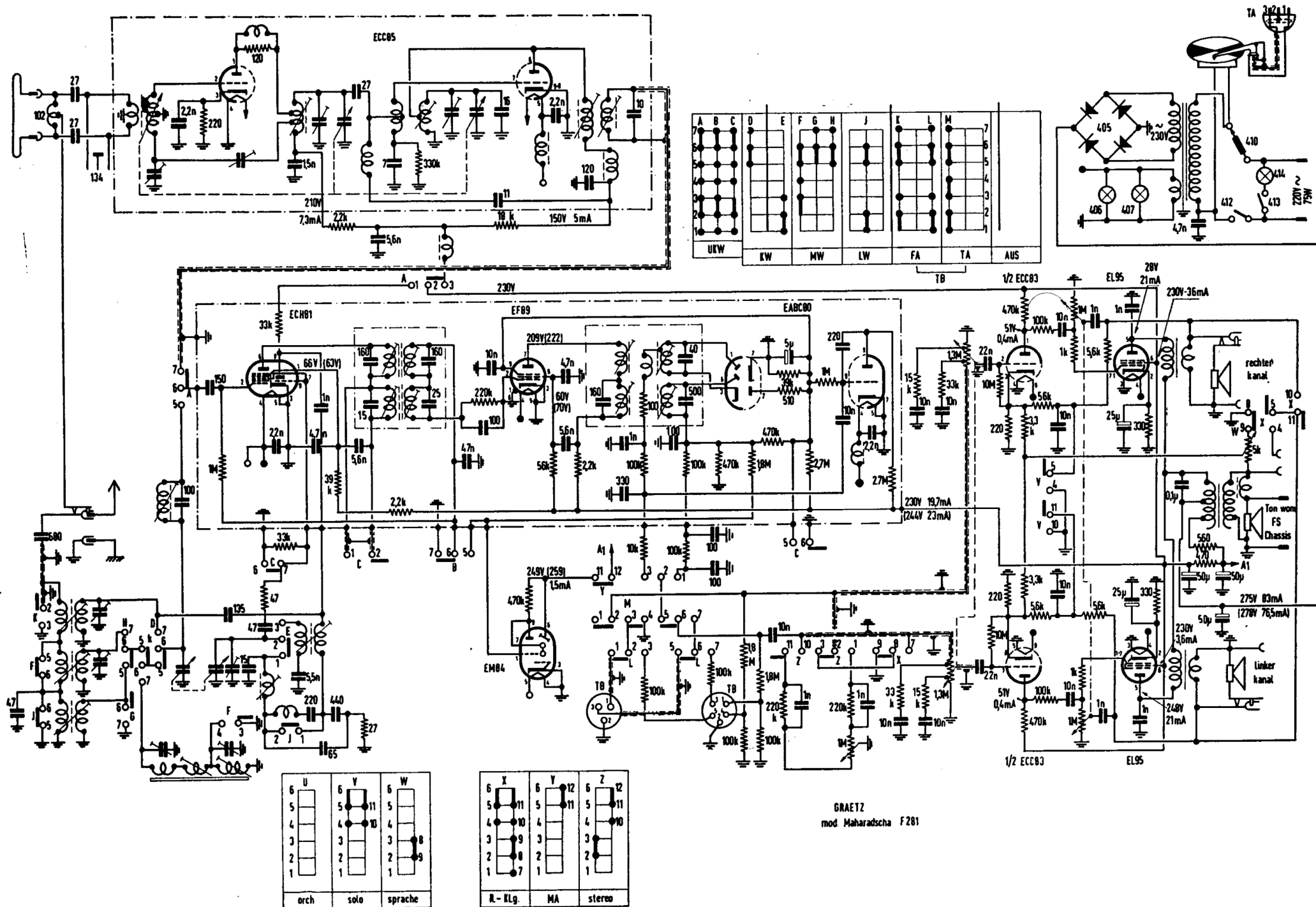
Schema elettrico del radiorecettore Graetz, mod. F 281
